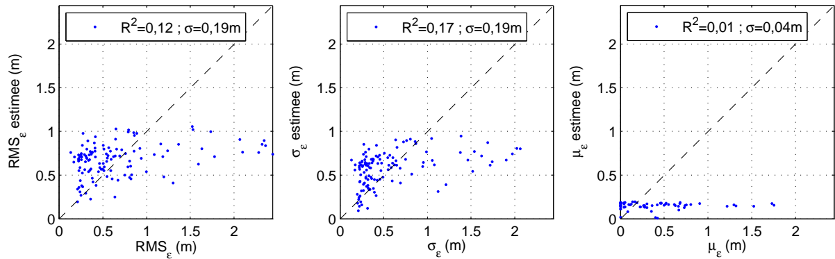
FIG. 8.7: Modèles saisonniers : Illustration de la sortie des modèles multivariables d'estimation des indicateurs de précision pour le produit alti-hydrologique RLH/ENVISAT en fonction de leurs valeurs réelles. La ligne en pointillé illustre la droite de corrélation idéale. Les valeurs de \sigma présentées dans les graphiques sont les écart-types de l'erreur résiduelle des modèles.
